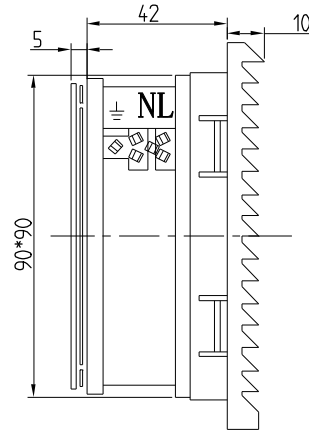
风扇及过滤器 FKL6621. 230 FKL6621. 115 FKL6621. 024 (包括 ①②③④ 零件)
