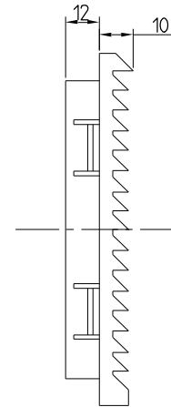
出口过滤器 FKL6621. 300 (包括 ①②④ 零件)
