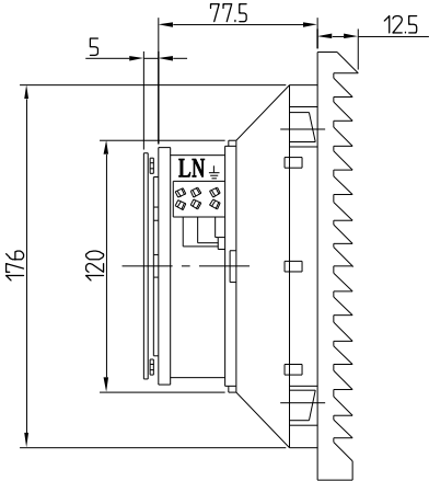
风扇及过滤器 FKL6623. 230 FKL6623. 115 FKL6623. 024 (包括 ①②④⑤ 零件)
