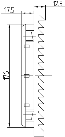
出口过滤器 FKL6623. 300 (包括 ①③⑤ 零件)
