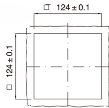
安装剖面 QR-3322
