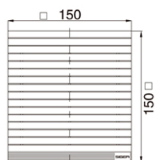
风扇及过滤器 QR-3322
