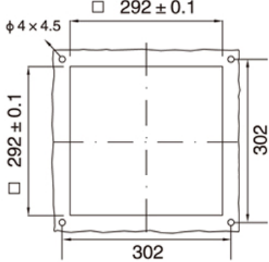
安装剖面 QR-3327
