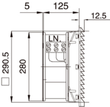
风扇及过滤器 QR-3327. 230
