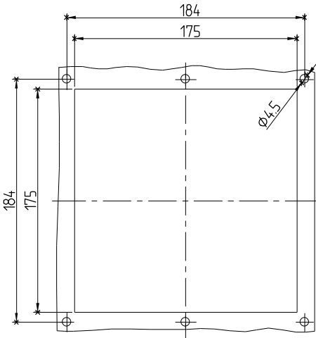
安装剖面 ZL-804
