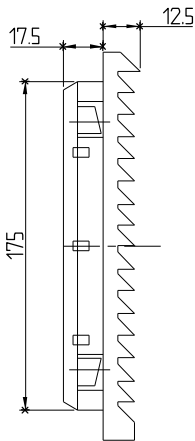
出口过滤器 ZL-804 (包括 ①③⑤ 零件)
