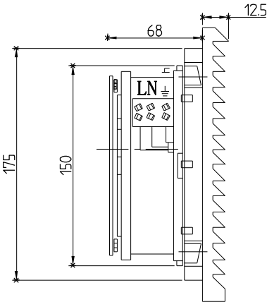
风扇及过滤器 ZL-804. 230 ZL-804. 115 ZL-804. 024 (包括 ①②④⑤ 零件)
