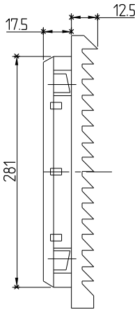
出口过滤器 ZL-806 (包括 ①③⑤ 零件)
