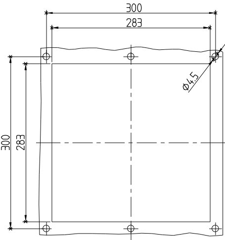
安装剖面 ZL-806
