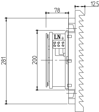
风扇及过滤器 ZL-806. 230 ZL-806. 115 (包括 ①②④⑤ 零件)
