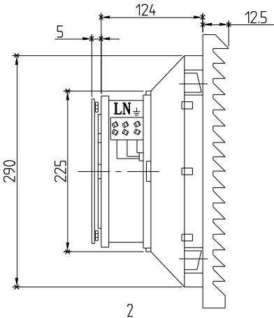
风扇及过滤器 CT320. 230 CT320. 115 (包括 ①②④⑤ 零件)
