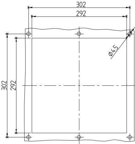
安装剖面 CT320....
