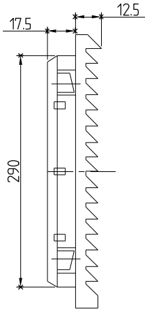
出口过滤器 CT320. 300 (包括 ①③⑤ 零件)
