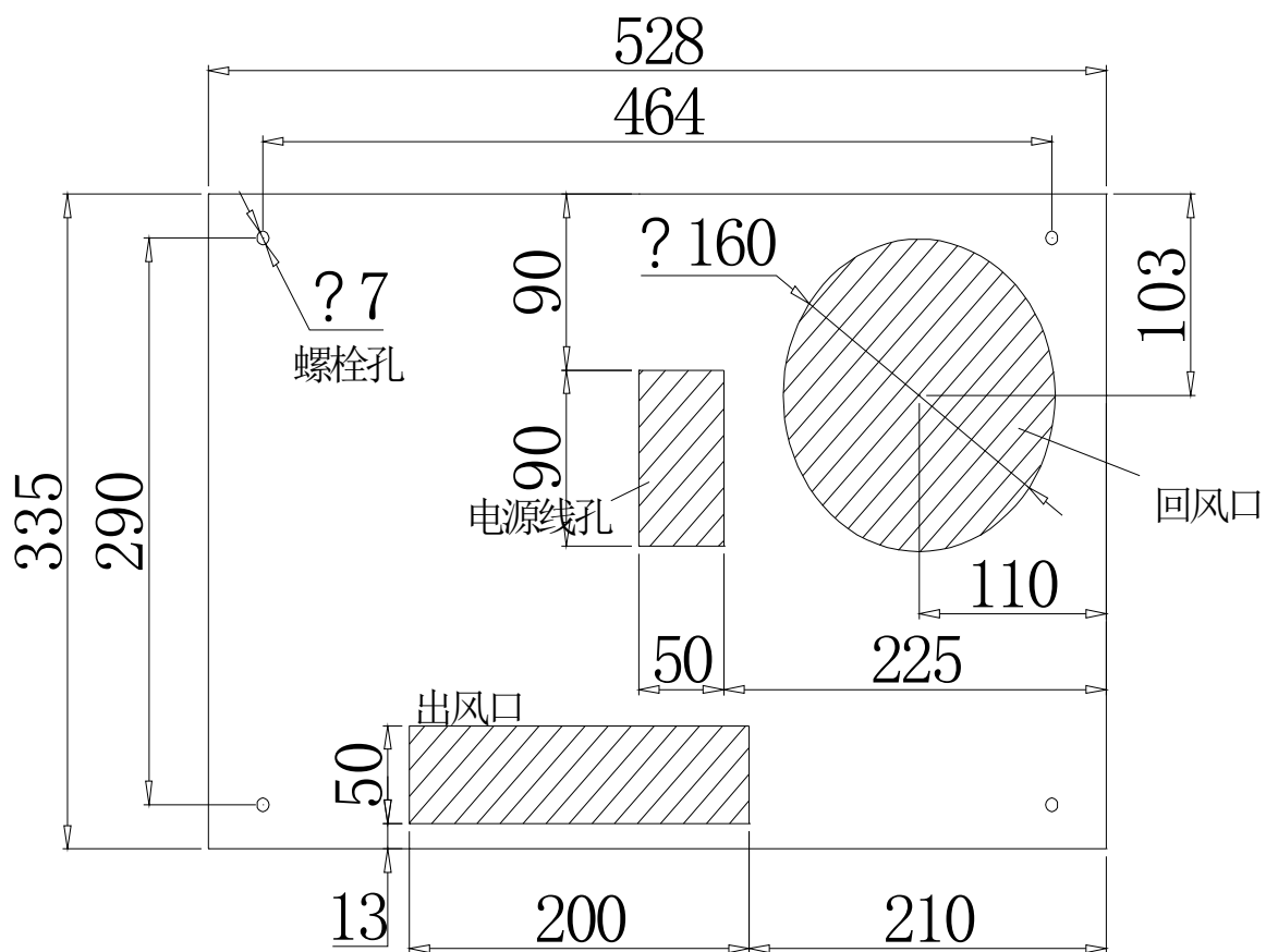
DEA-800 开孔图 (阴影部分开孔)
